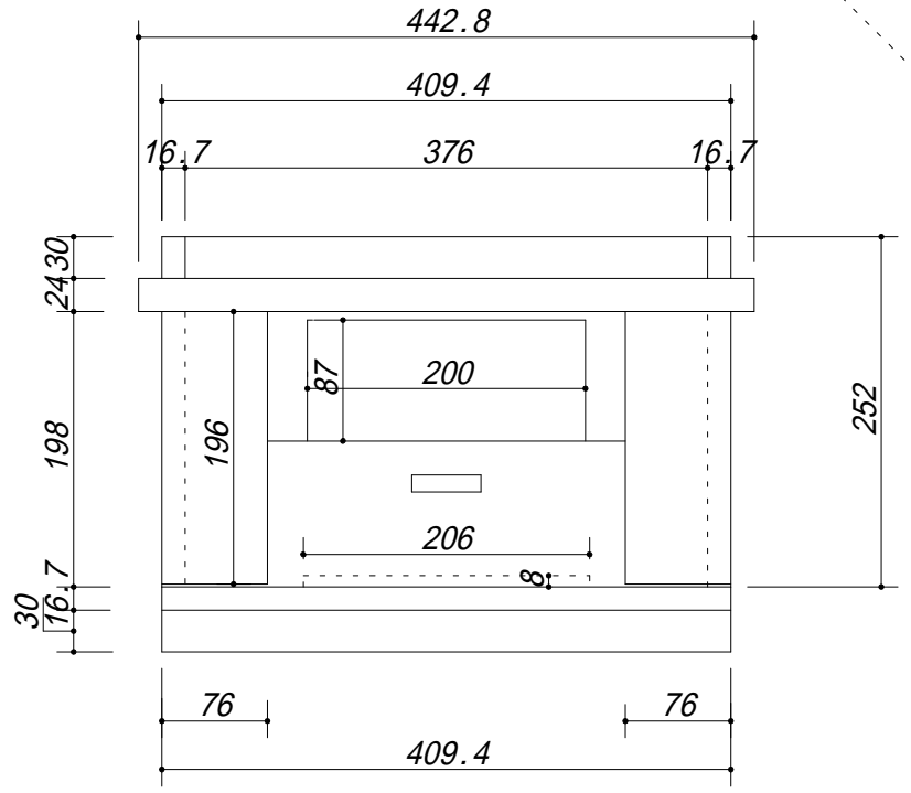
本体正面
