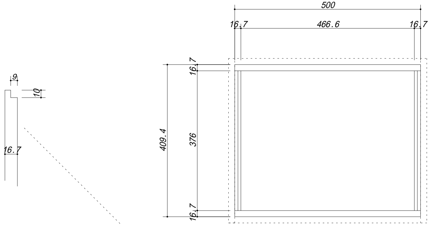
本体正面
