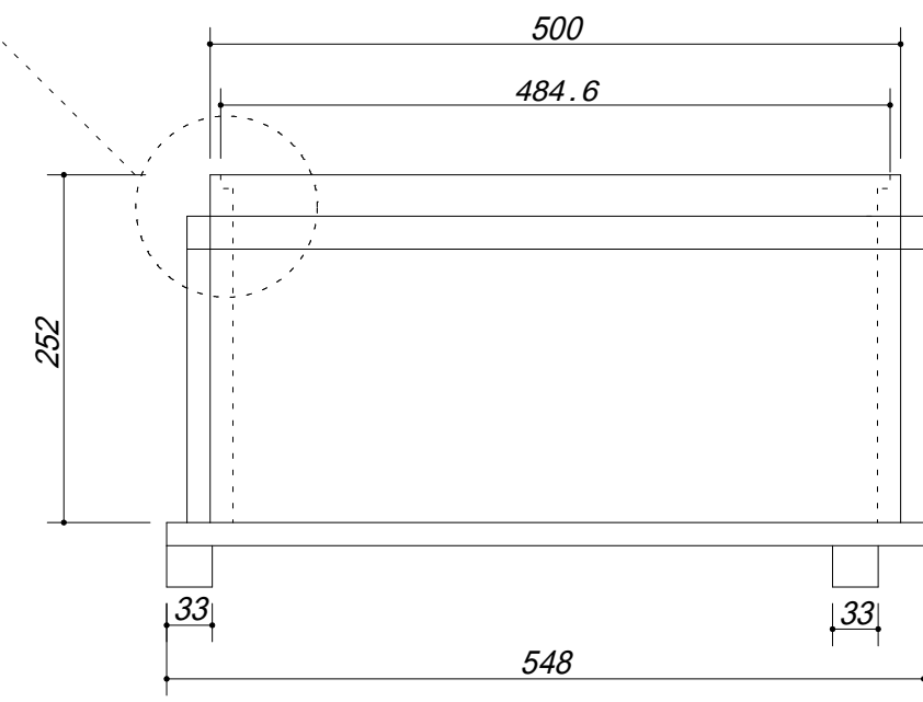
本体側面
