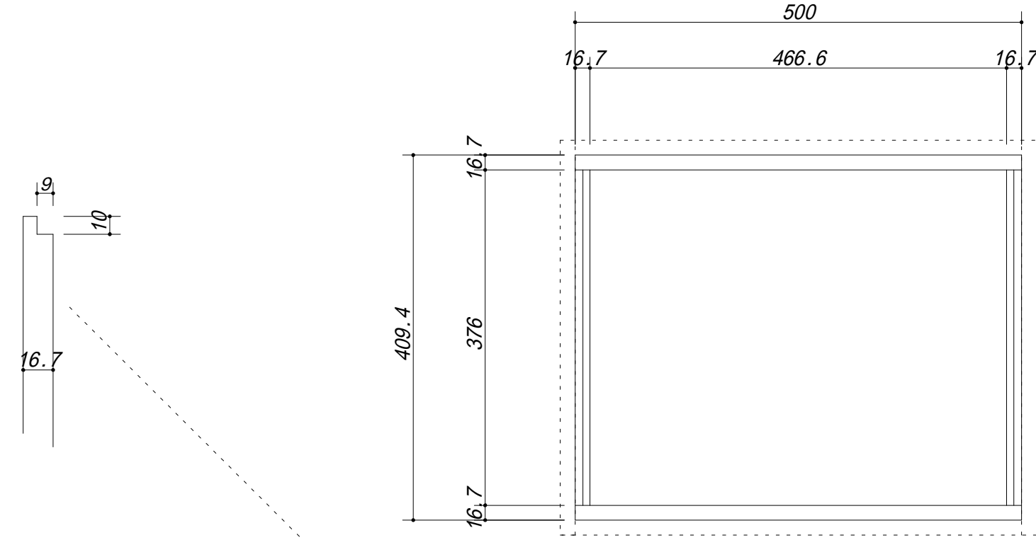
本体正面
