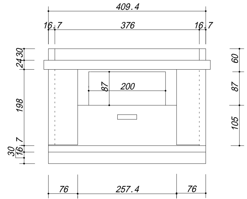
本体裏面
