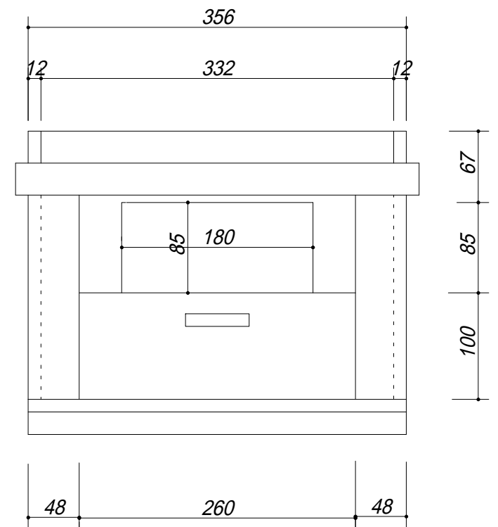
本体裏面
