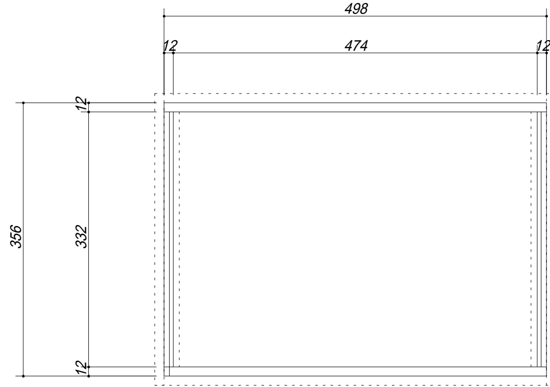
本体側面
