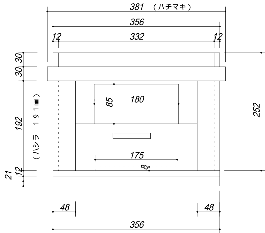
本体正面
