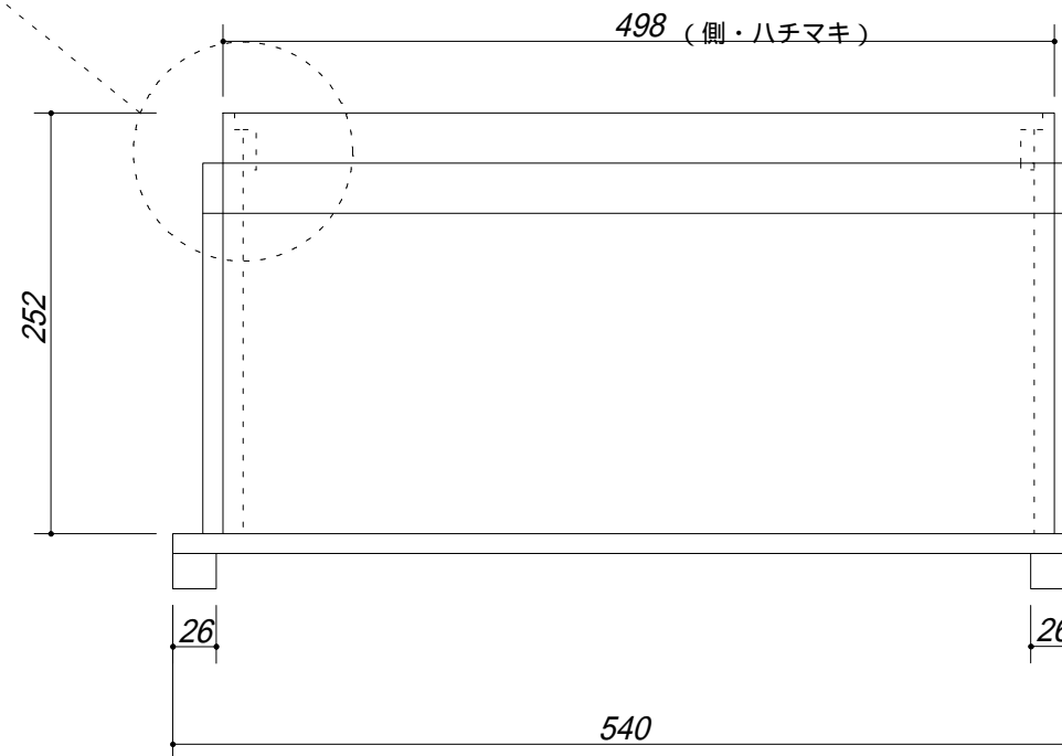
本体側面
